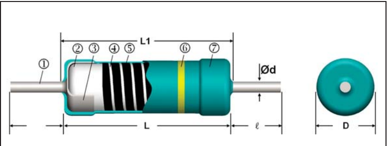
結構圖 Construction
